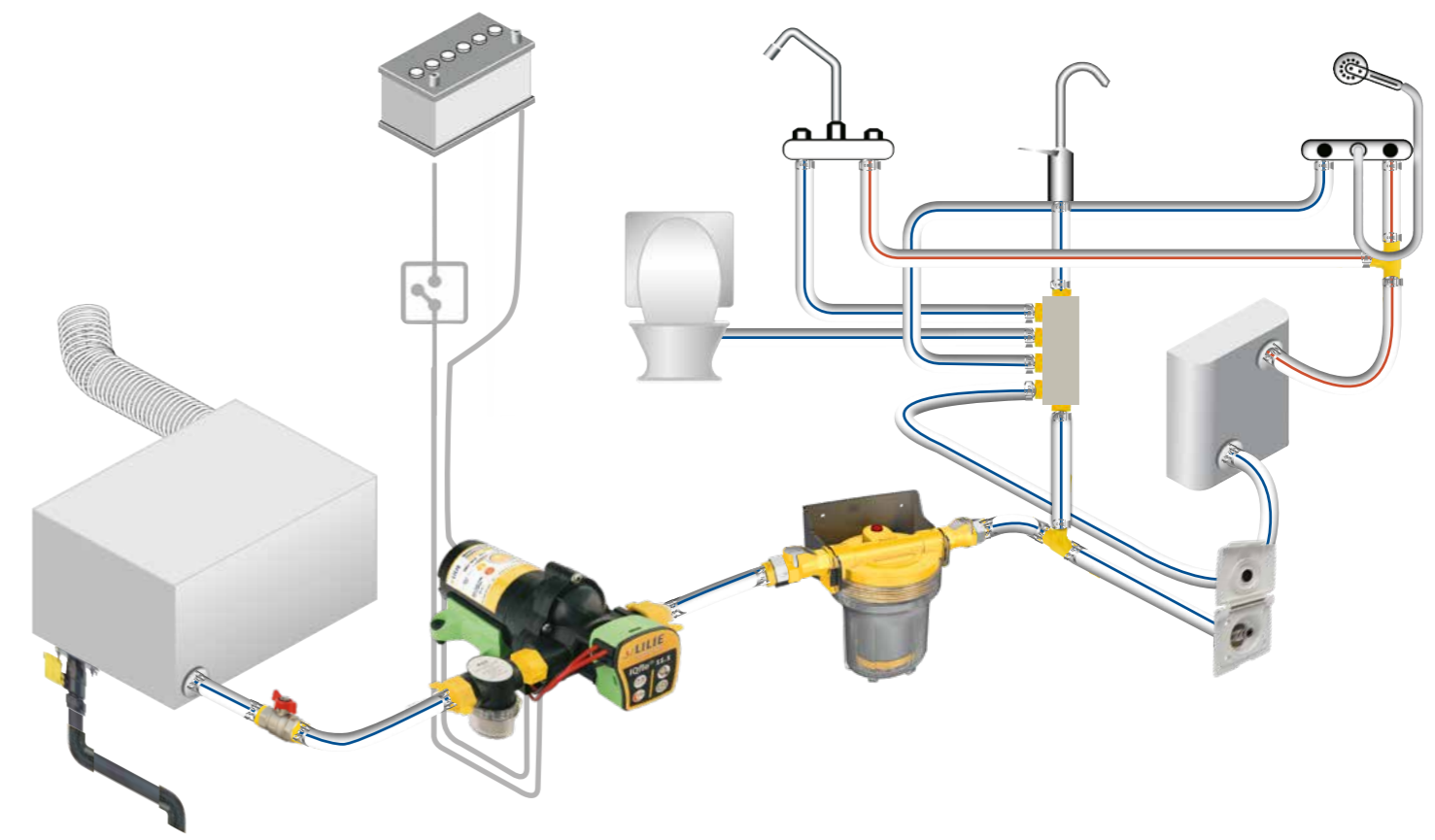
BEISPIEL EINES TRINKWASSERSYSTEMS GEM. DIN 2001-2 IM BEREICH CARAVANING.
